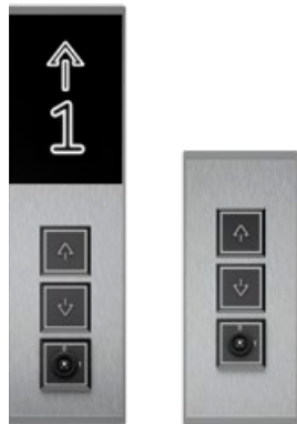
Landing Operating Panels HALO SL631 DIMENSIONS WITH DISPLAY (W) 95 mm x (D) 14 mm x (H) 335 mm HALO SL630 DIMENSIONS WITHOUT DISPLAY (W) 95 mm x (D) 14 mm x (H) 225 mm
